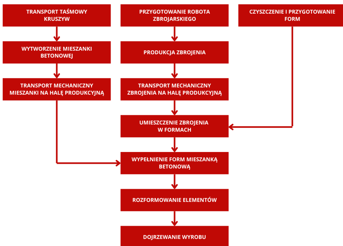
Rysunek 5.2: Schemat procesu produkcji prefabrykowanych pali żelbetowych w Centrum Pali Sp. z o. o. .
