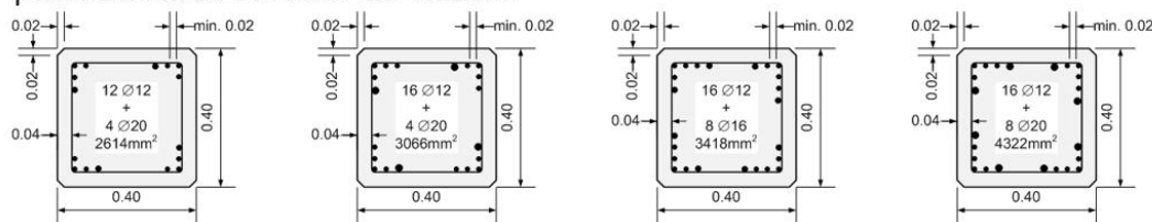
Rysunek 4.2: Warianty średnicy i układu prętów
